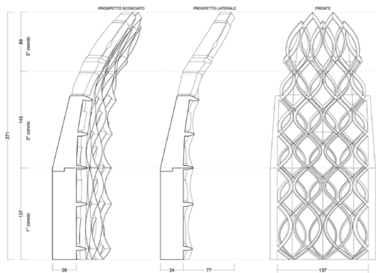
Fig. 4. Cirillo e Metodio's Dome (Claudio D'Amato, Giuseppe Fallacara, Graziella Fittipaldi, Francesco Scricco, 2012).
