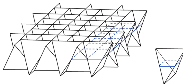
Fig. 1. Dettaglio di un gruppo piano di tetraedri topologicamente interbloccati.
