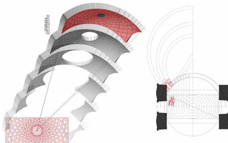
Fig. 13. Rapporto tra apparecchiatura di tipo conico e trama decorativa 14 .
