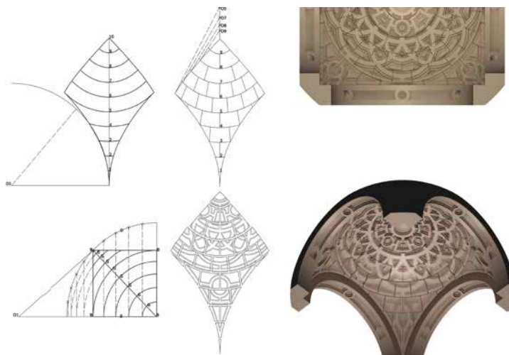
Fig. 15. Alonso de Vandelvira, Capilla Enlazada 115v.
